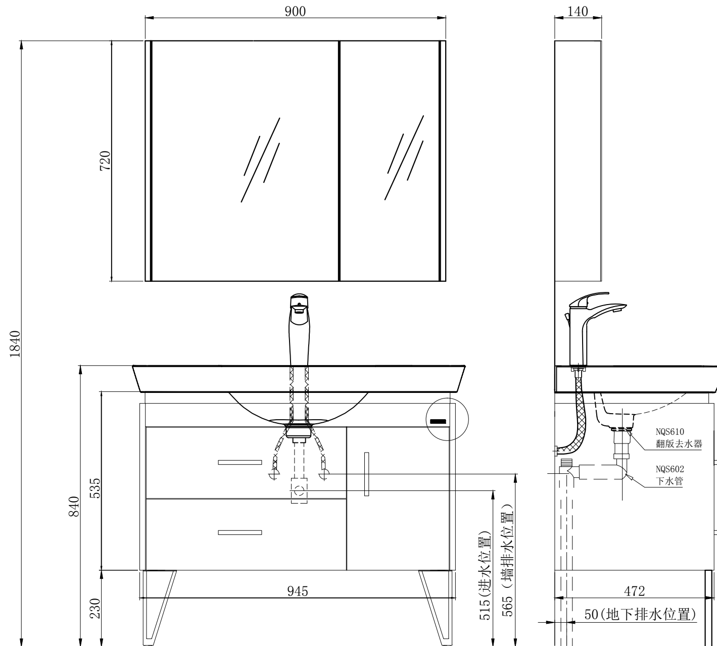
N1D10G07 生态实木柜水电安装图（建议安装尺寸）
