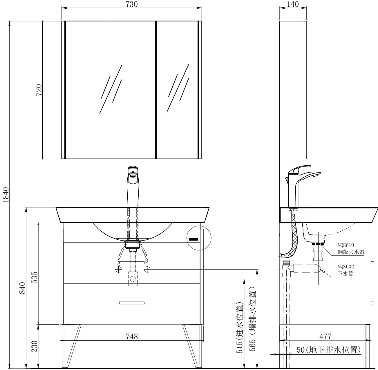
N1D80G07 生态实木柜水电安装图（建议安装尺寸）
